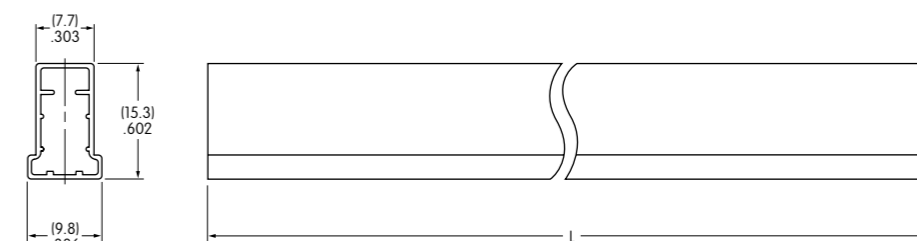
粘贴管尺寸
